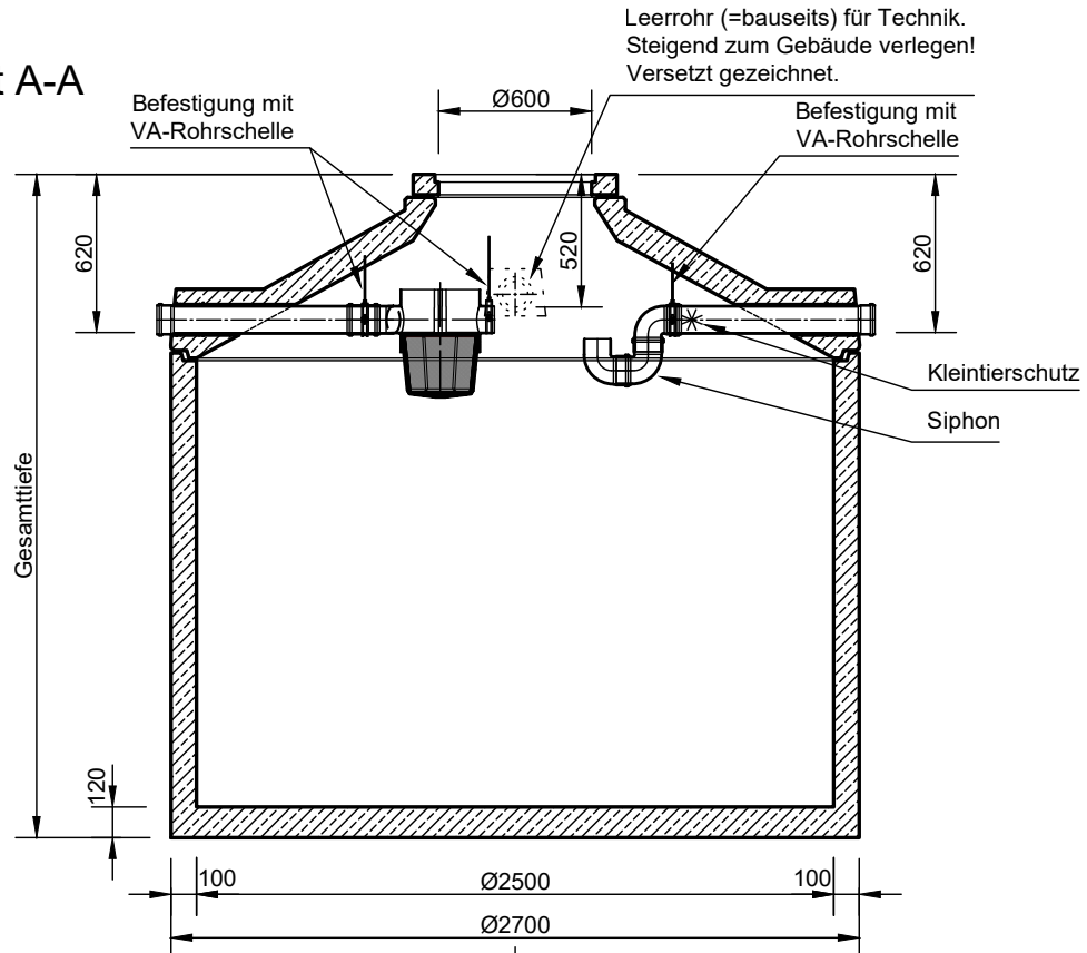
Grundriss
